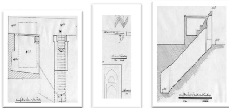
نقشه ۱. پلان آب انبار محمد صالح بیگ.
